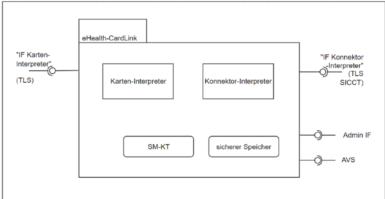
Abb. 2: Produktzerlegung eH-CL
